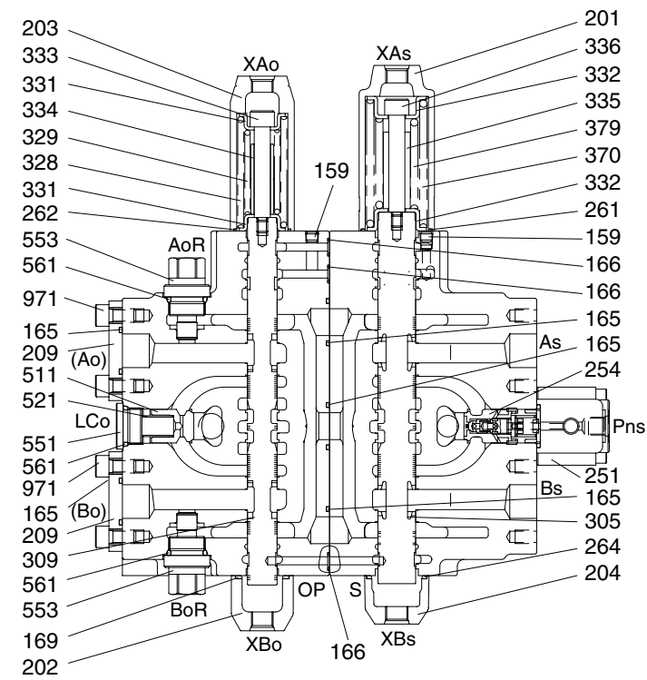
SECTION D-D
