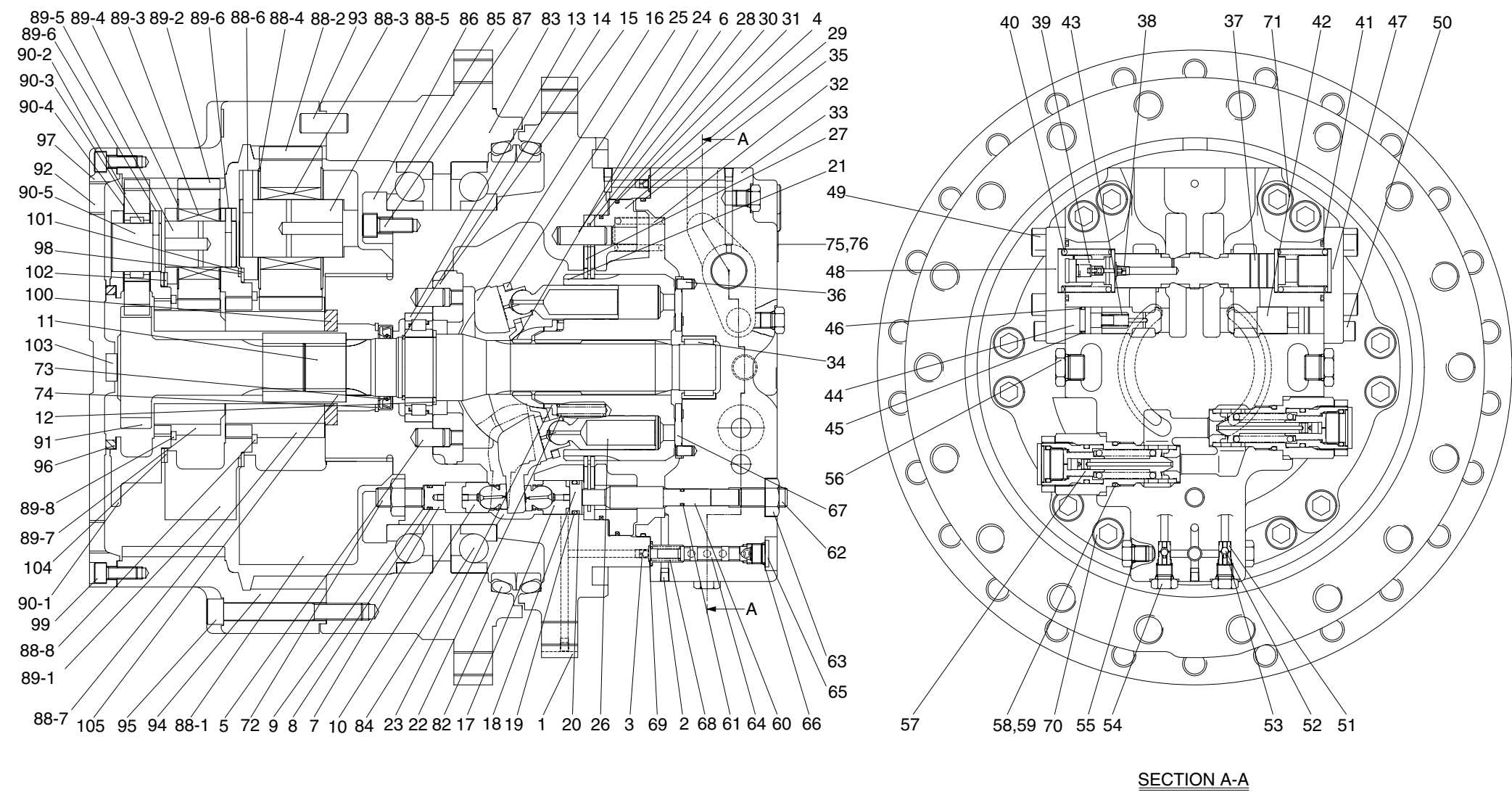
SECTION A-A
