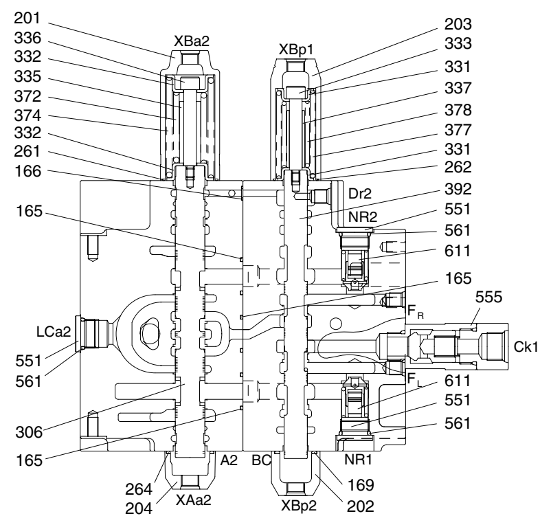
SECTION D-D
