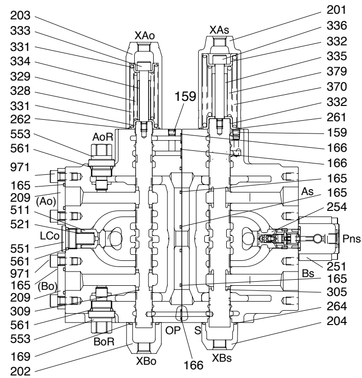
SECTION D-D
