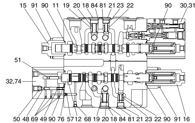
E - E (ARM 1 & ARM REGENERATION /BREAKER)
